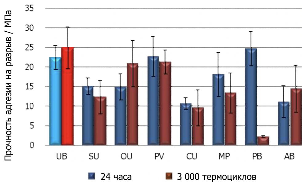
Рис. 37 Прочность адгезии (на разрыв) композитных цемента к эмали до и после циклического термического воздействия
