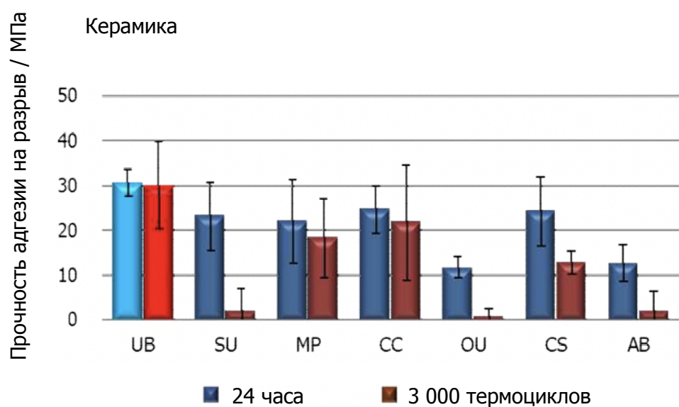
Рис. 43 Прочность адгезии на разрыв при использовании Tokuyama Universal Bond II и праймеров для керамики
