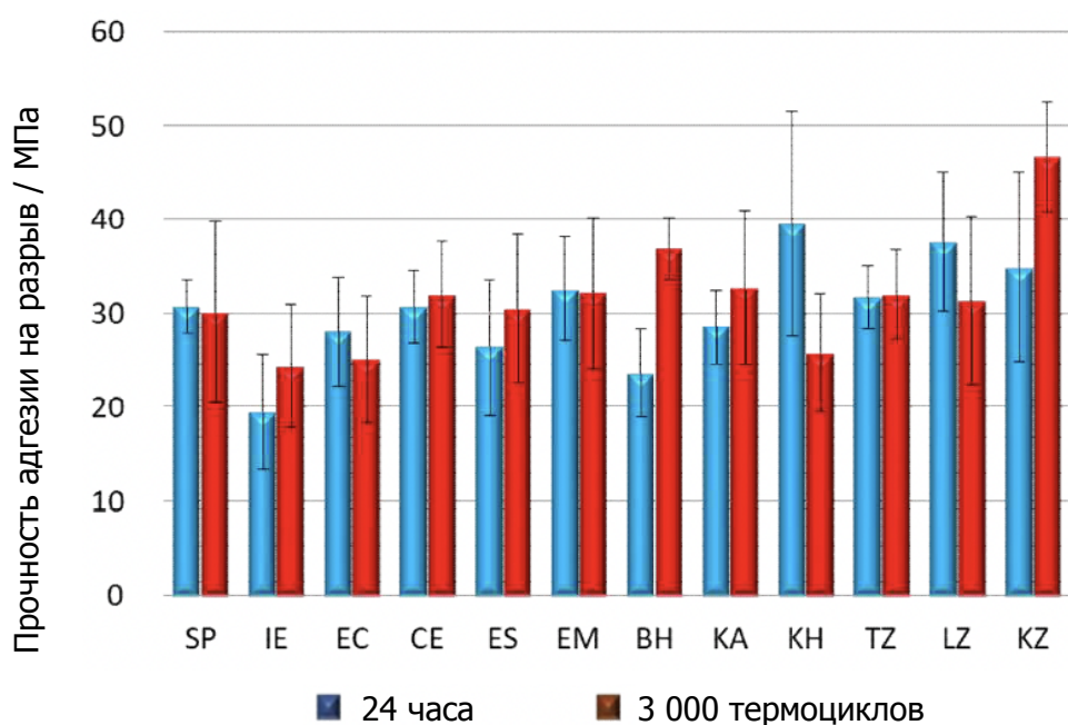
Рис. 40 Прочность адгезии на разрыв к керамике, непрямому композиту, CAD/CAM-блокам и оксиду циркония при использовании Tokuyama Universal Bond II
