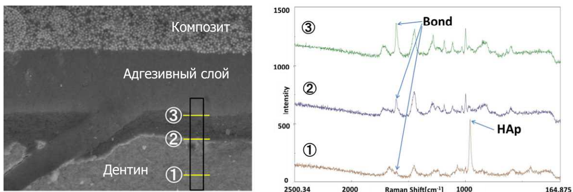
Рис. 24 Рамановская спектроскопия Tokuyama Universal Bond II
