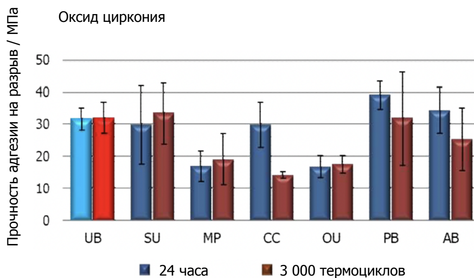
Рис. 45 Прочность адгезии на разрыв при использовании Tokuyama Universal Bond II и праймеров для оксида циркония
