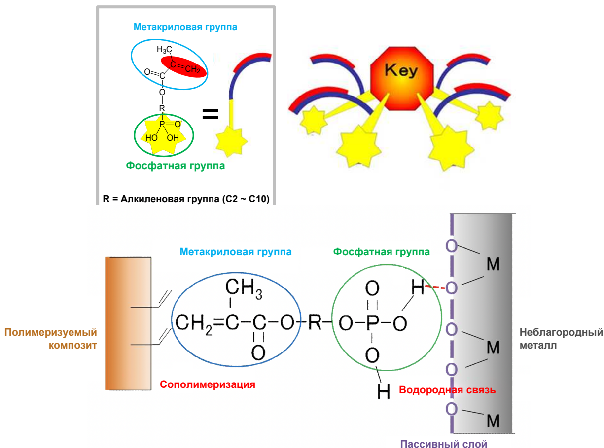
Рис. 6 Механизм адгезии к неблагородным металлам (схематически) 6,9)
