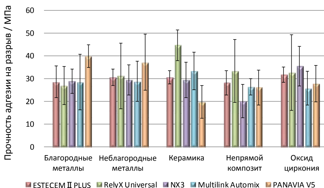
Рис. 46 Сравнительная прочность адгезии к реставрационным материалам при использовании разных композитных цемента
