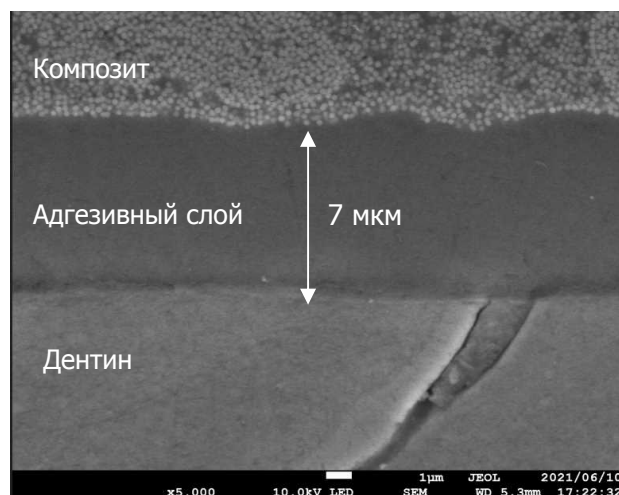
Рис. 22 Дентин (x 5 000)
